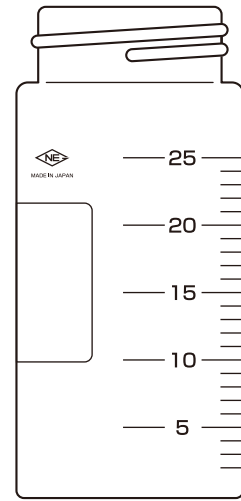
GV-25 (30 x 65)
